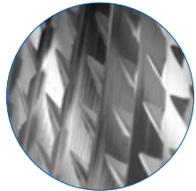
Kreuzverzahnung mit Querhieb
